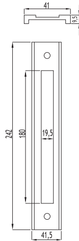
02 - 016 C60 Kilit Altı C60 Under Lock
