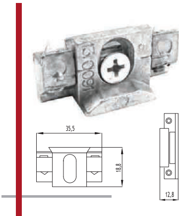
02 - 017 Ayarlı İspanyolet Set Spaniard
