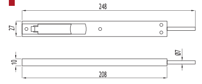
02 - 023 Sistem Kısa Sürgü System Short Latch
