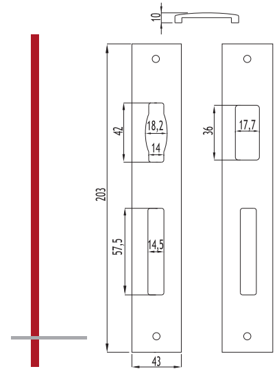
02 - 017 C60 Elektrikli Kilit Altı C60 Under Lock
