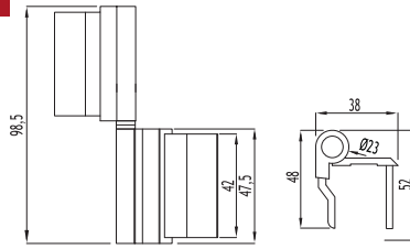
02 - 004 A Sistem Menteşe Tip - 2 System Hinge Type 2
