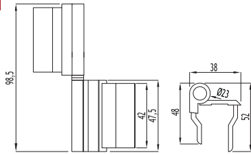
02 - 004 Sistem Menteşe System Hinge
