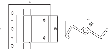
02 - 009 Alüminyum Yaylı Menteşe Aluminium Spring Hinge
