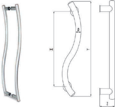
S Kol Pull Door Handle S Type
