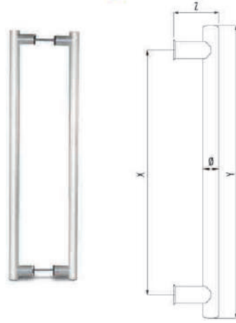
H Kol Pull Door Handle H Type
