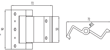
02 - 006 Pivot Menteşe Pivot Hinge
