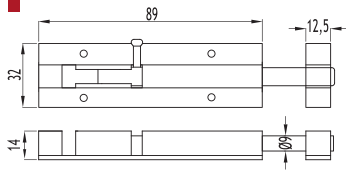
02 - 024 Sistem Uzun Sürgü (Dar) System Long Latch (Narrow)
